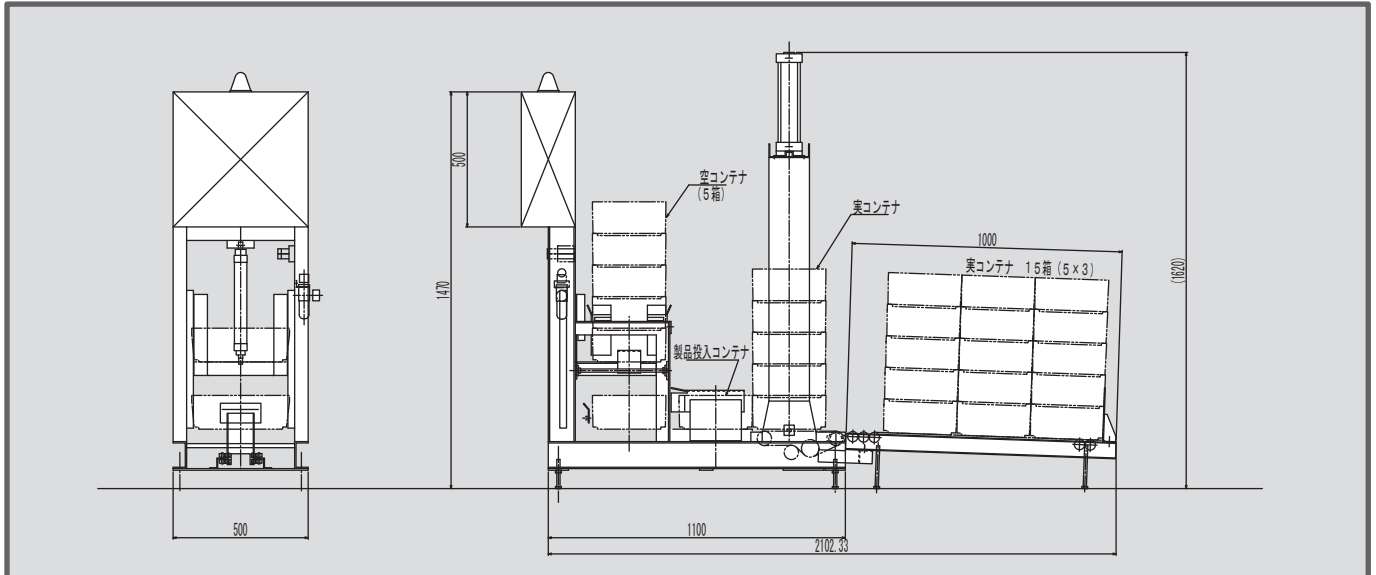
タテ・タテタイプ外観寸法
